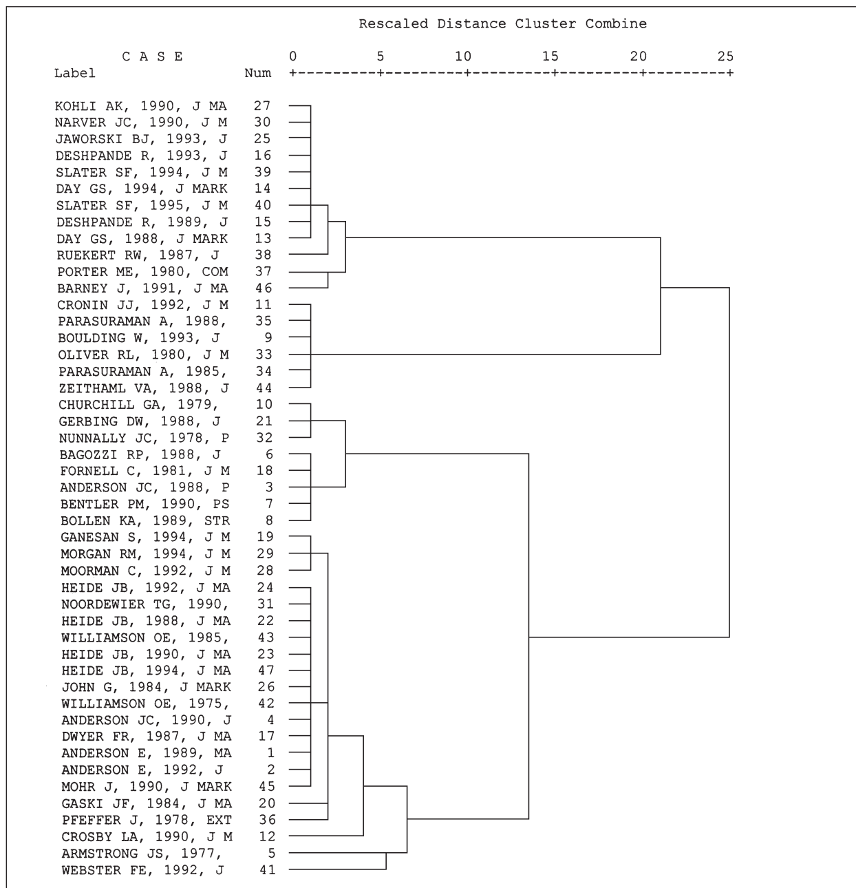
FIGURA 1 Dendrograma
